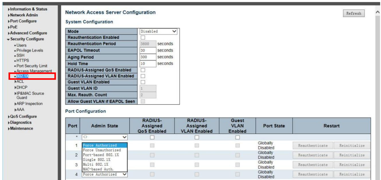
Рисунок 7-7 Экран конфигурации системы аутентификации IEEE 802.1X
