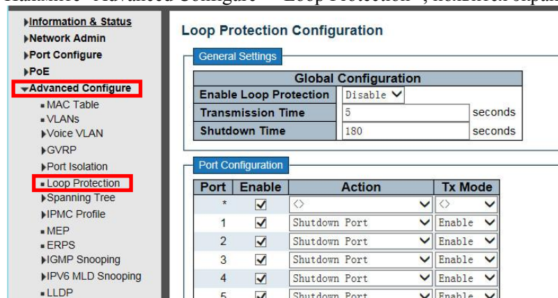
Рисунок 5-9 Экран настройки защиты от петель
