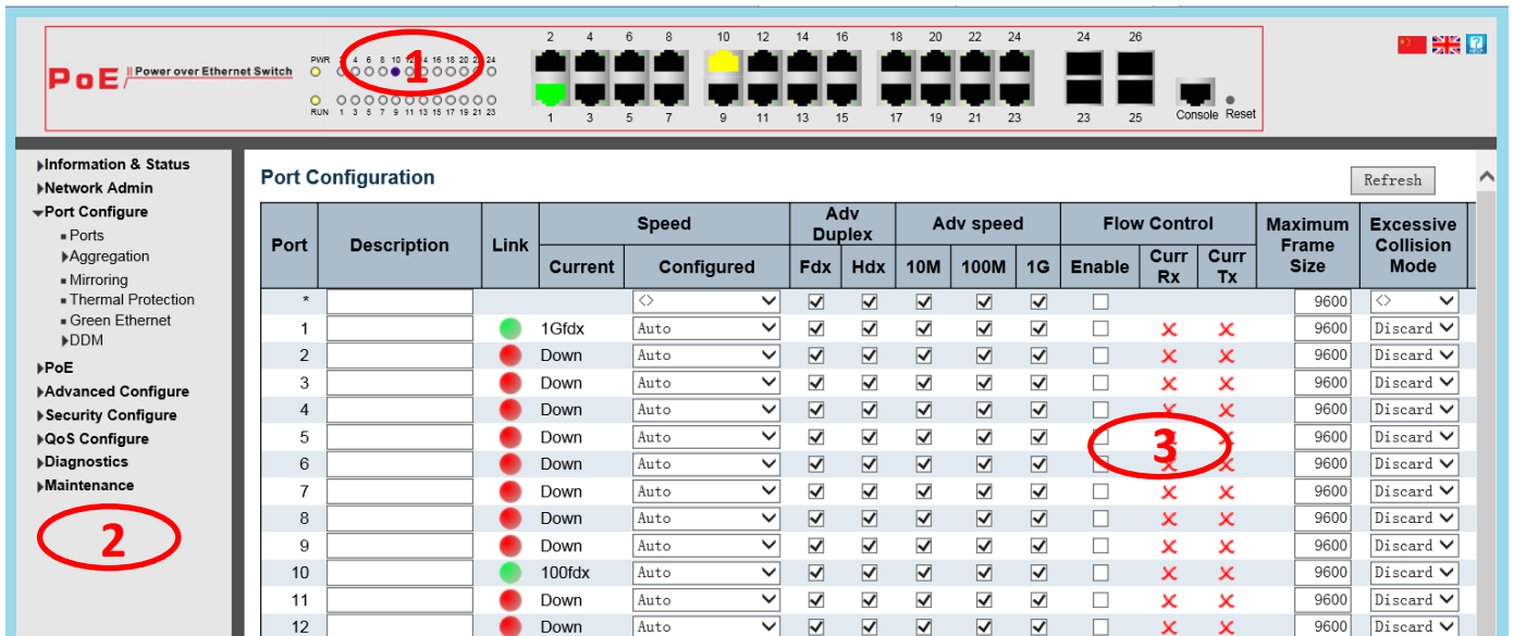
Рисунок 1-2 Интерфейс главной страницы веб-управления
