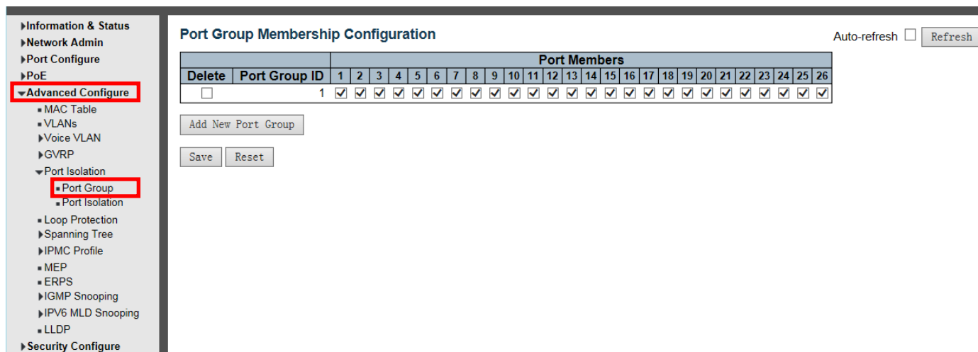
Рисунок 5-2-1 Экран конфигурации группы портов
